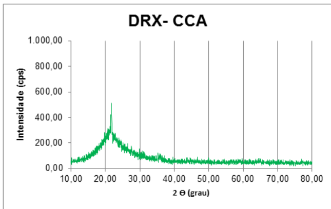
Fig. 3. Difração de Raios X da Cinza de Casca de Arroz
