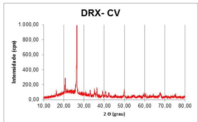
Fig. 2. Difração de Raios X da Cinza Volante
