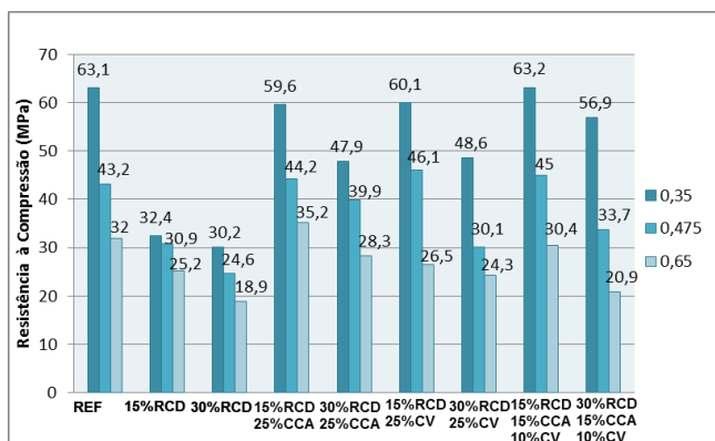
Fig. 4. Resistência à Compressão Axial de todas as misturas estudadas
